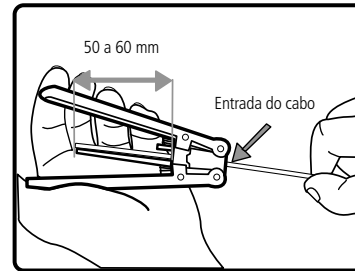
1. Retire a capa do cabo Drop
