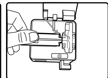
8. Corte a fibra
