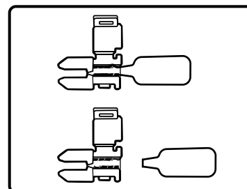
5. Se estiver utilizando um cabo drop 1 indoor (1,6×2 mm), engate o suporte plástico que acompanha o produto dentro do grampo e quebre a parte externa.
