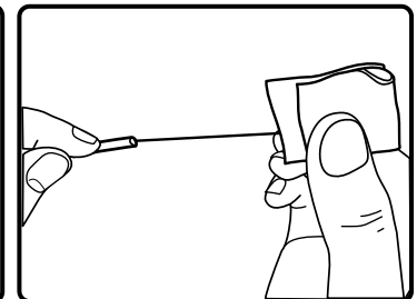
4. Limpe a fibra óptica com o lenço umedecido com álcool isopropílico
