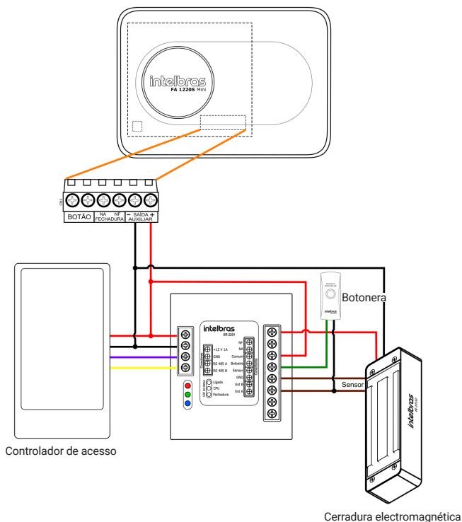
Esquema de liqación con XR 2201
