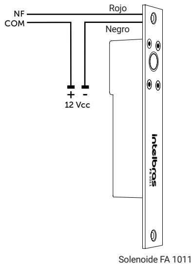
Ejemplo de conexión de cerradura de solenoide FA 1011
