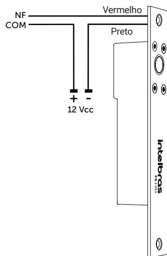
Solenoide FA 1011
