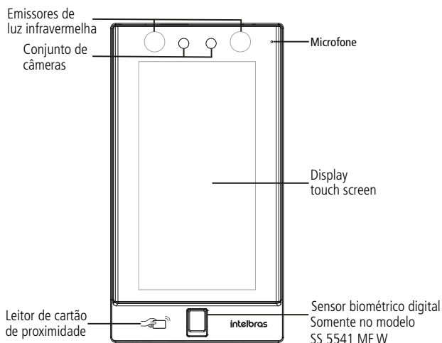
Visão frontal SS 5541 MF W
