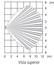
Vista superior
