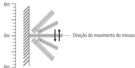
Vista superior
