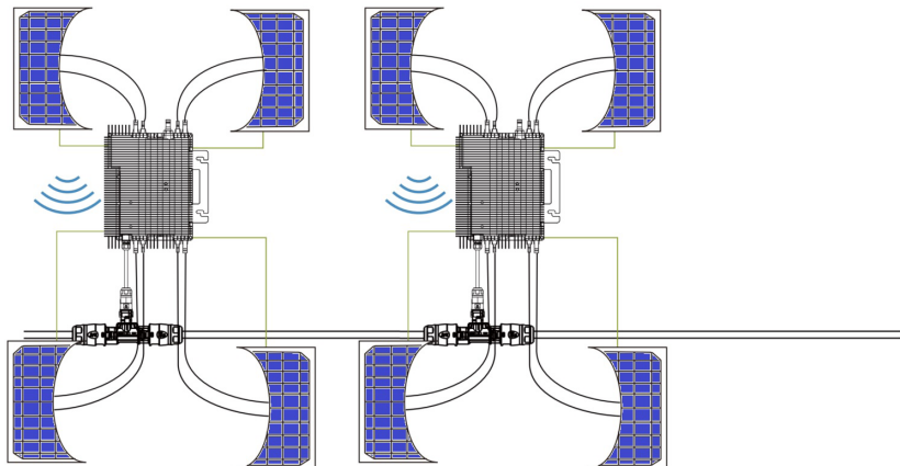
Microinversores conectados em paralelo
