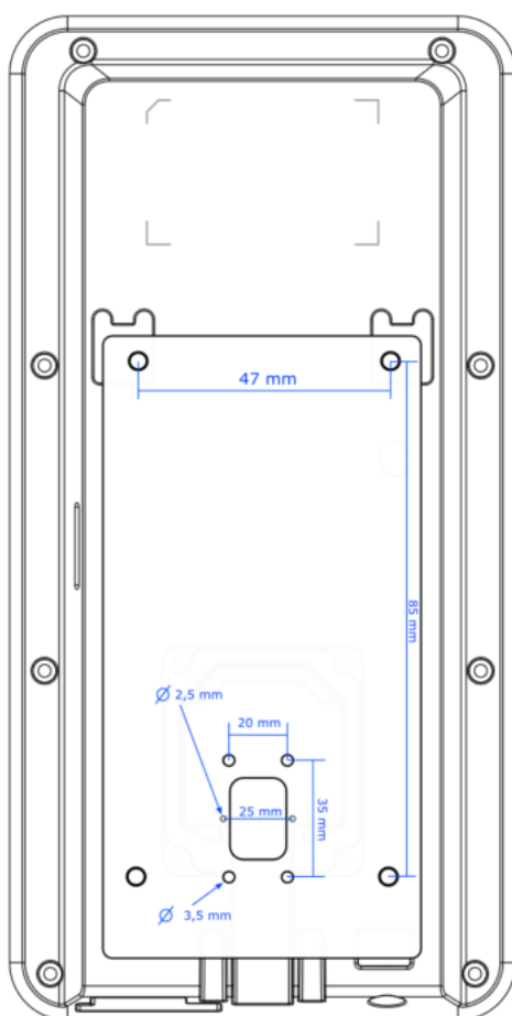
Gabarito de furação
