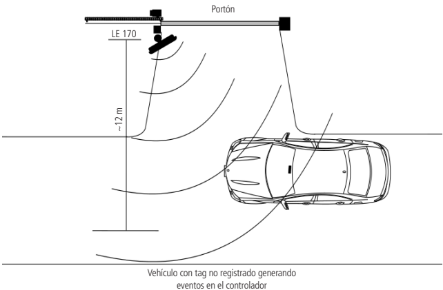
Ejemplo con ajuste de potencia máxima (30)
