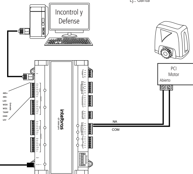
Conexión CT 3000 con cable manga blindado
