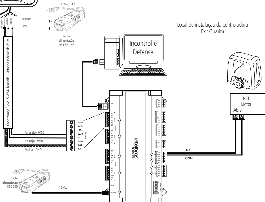
Ligação CT 3000 com cabo mangá blindado
