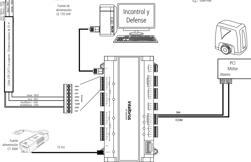
Conexión CT 3000 con cable UTP
