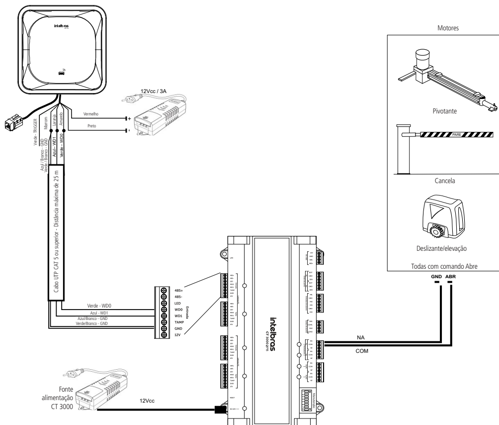
Acionamento placa acionadora com comando ABR
