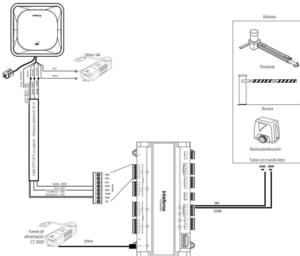
Accionamiento placa accionadora con mando ABR
