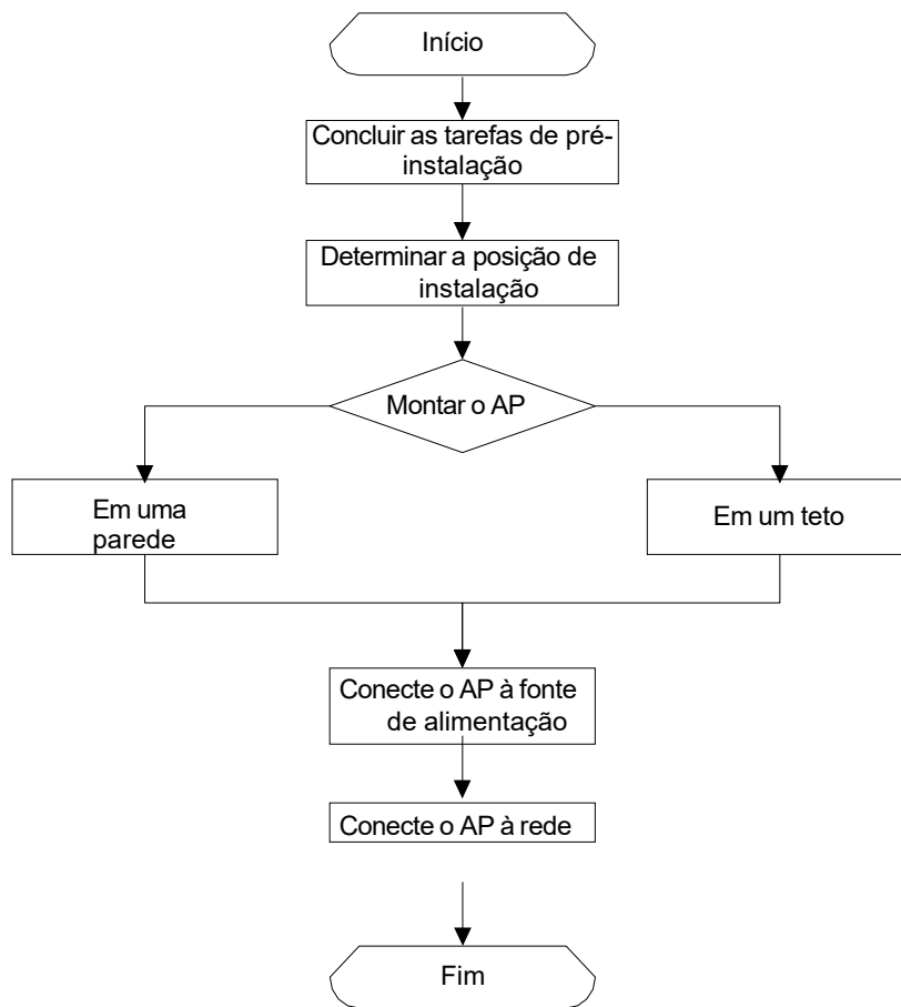
Figura 2-1 Fluxograma de instalação
