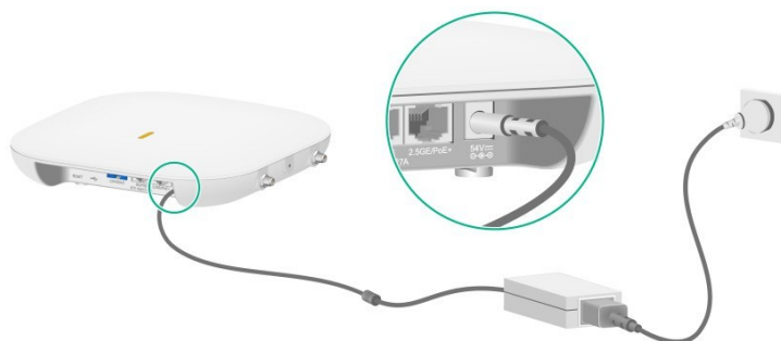
Figura 2-15 Uso de um adaptador de energia para conectar o AP a uma fonte de energia local
