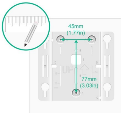
Figura 2-4 Marcação dos orifícios de instalação na parede
