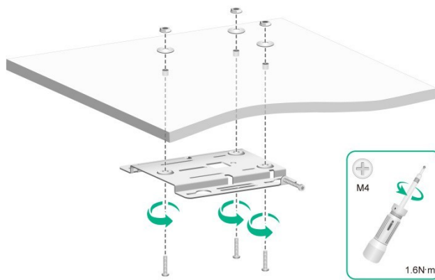
Figura 2-12 Fixação do suporte de montagem no teto
