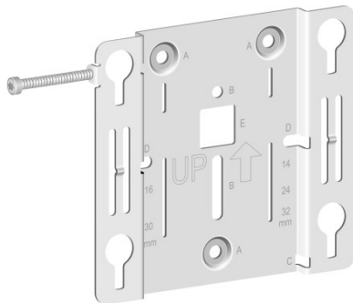
Figura 2-7 Inserção do parafuso de segurança
