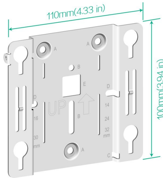
Figura 2-3 Dimensões do suporte de montagem
