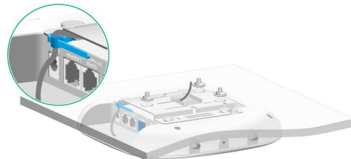
Figura 2-14 Uso de uma braçadeira para prender o cabo
