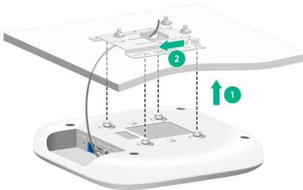
Figura 2-13 Fixação do AP no suporte de montagem
