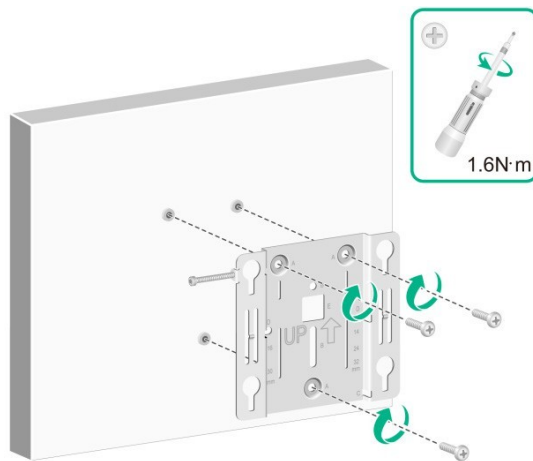
Figura 2-8 Fixação do suporte de montagem na parede
