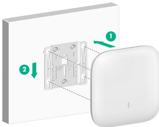
Figura 2-9 Fixação do AP no suporte de montagem
