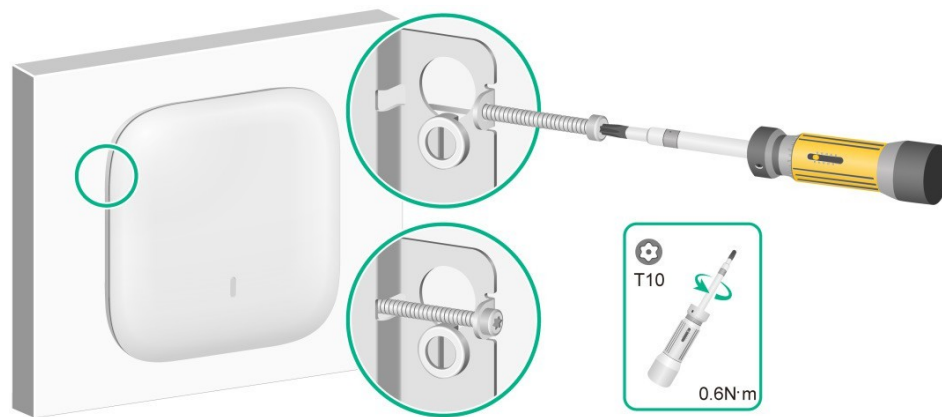
Figura 2-10 Fixação do parafuso de segurança M3 × 23,5
