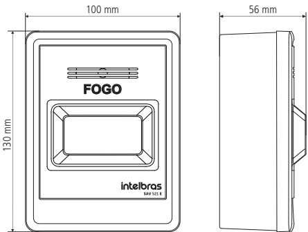
Vista frontal e lateral
