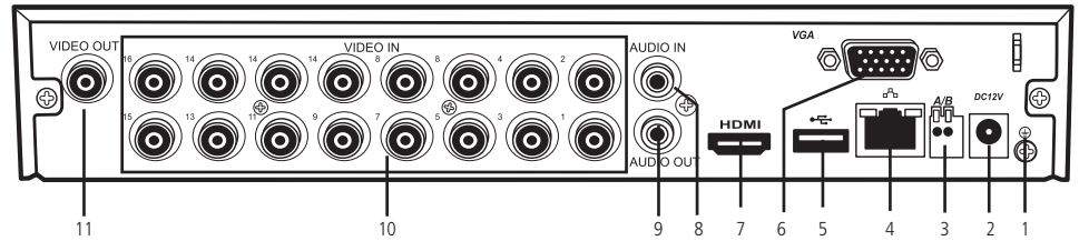
Painel posterior
