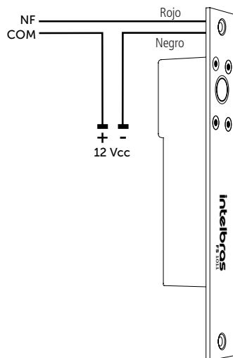
Solenoide FS 1011
