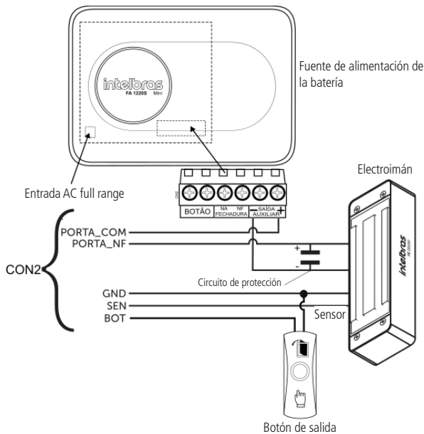
Ejemplo de conexión de cerradura electroimán con sensor
