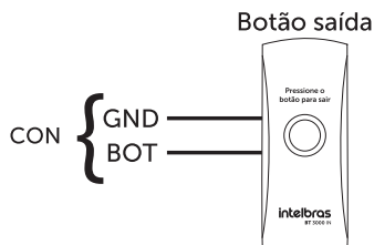
Exemplo de ligação de botão de saída
