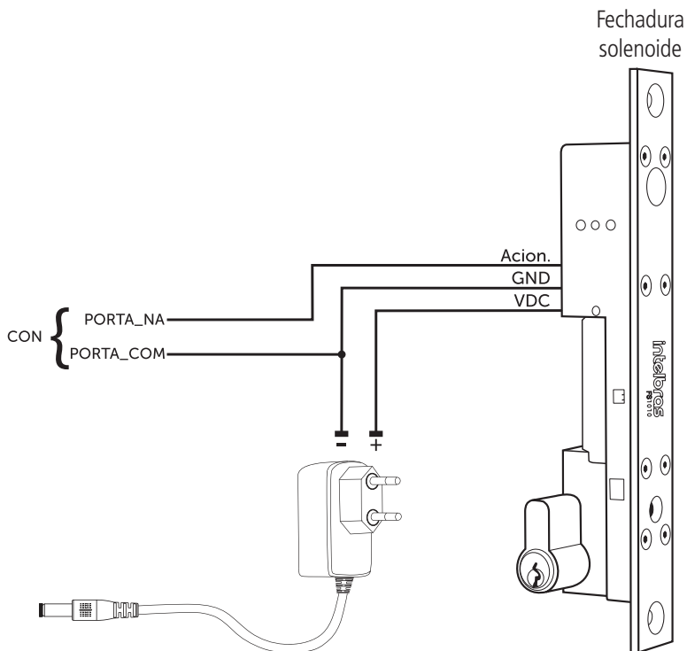
Ejemplo de conexión de cerradura de solenoide FS 1010
