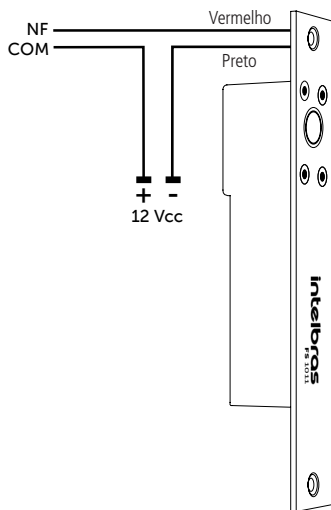
Solenoide FS 1011
