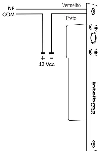
Solenoide FS 1011
