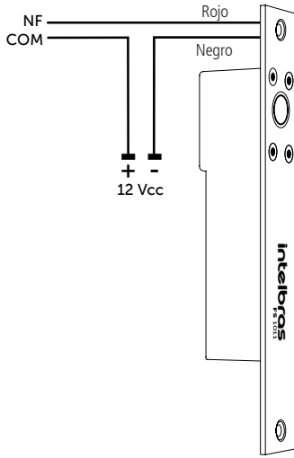
Solenoide FS 1011
