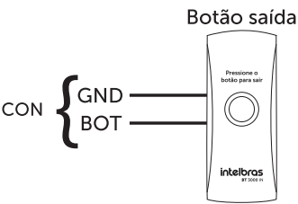
Exemplo de ligação de botão de saída
