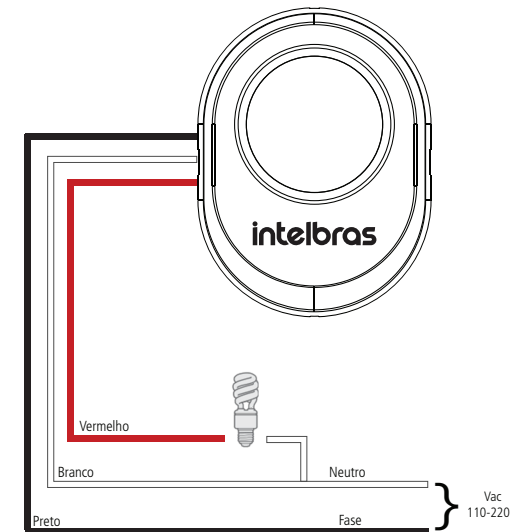
Conexões elétricas
