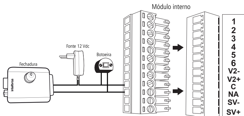
Instalação da fechadura no modo seguro
