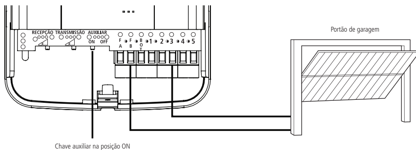
Instalação do portão de garagem
