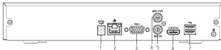
Painel posterior
