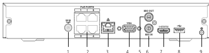
Painel posterior NVD 3204 P
