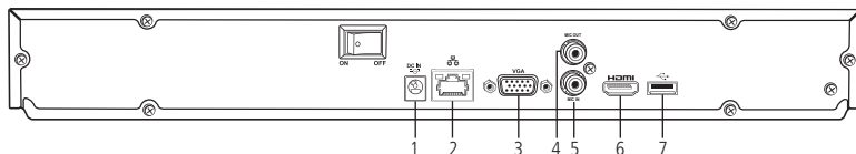
Painel posterior
