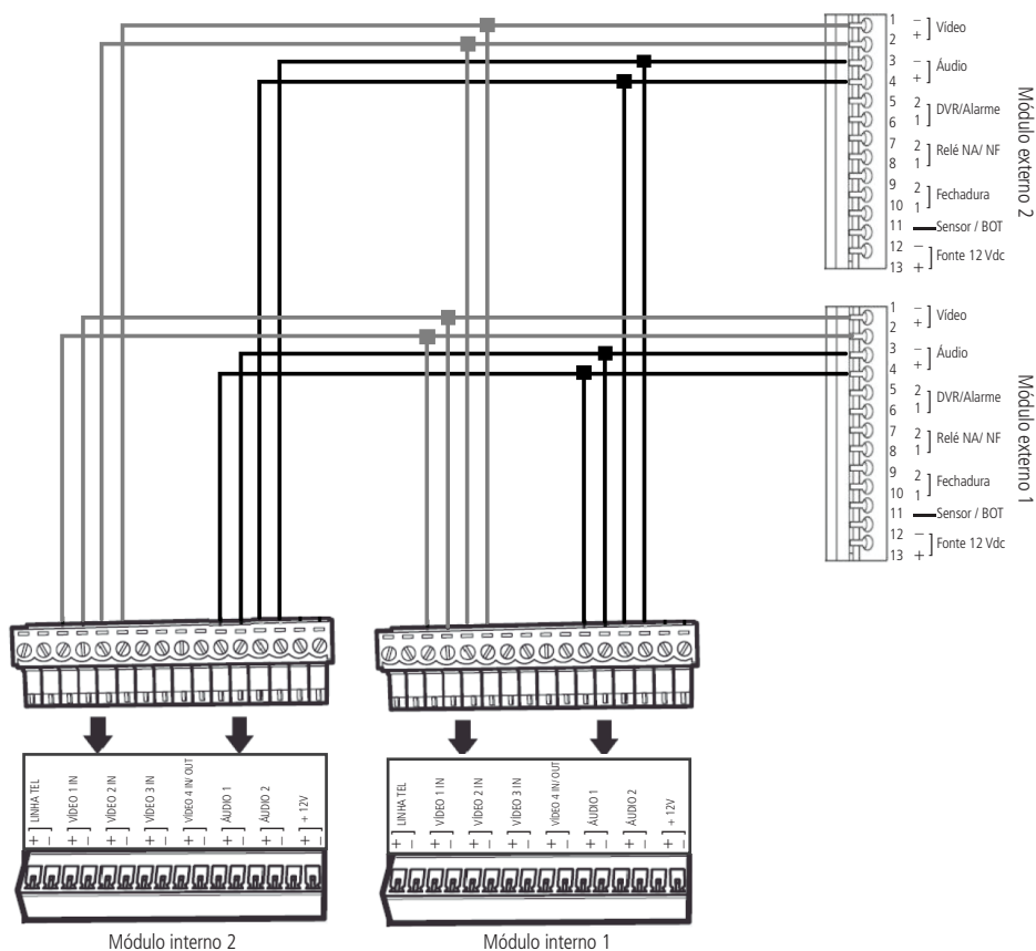
Conexão 2 módulos internos e 2 módulos externos
