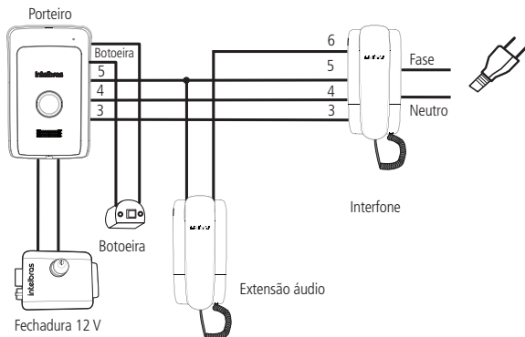
Exemplo 1 – ligação do porteiro e periféricos utilizando fechadura elétrica e botoeira
