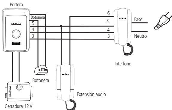
Ejemplo 1— conexión del portero y periféricos utilizando cerradura eléctrica y botonera
