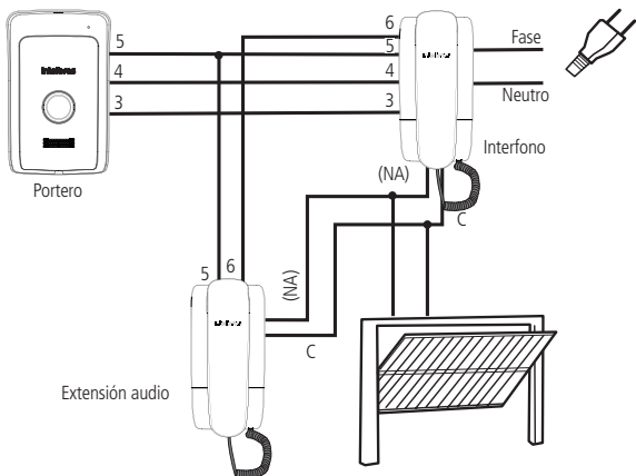
Ejemplo 2— conexión del portero y periféricos utilizando portón a motor
