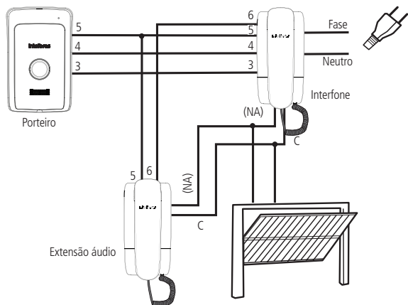
Exemplo 2 – ligação do porteiro e periféricos utilizando portão a motor
