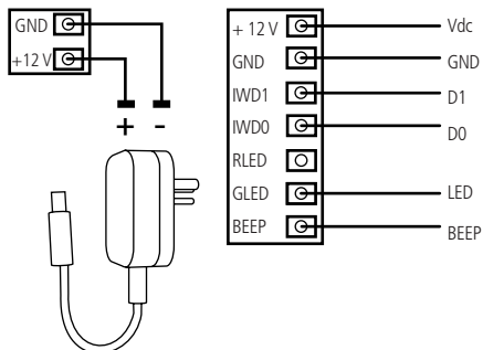
Fonte de alimentação
