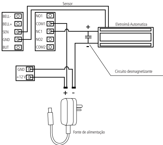
Ligação fechadura-eletoímã Automatiza
