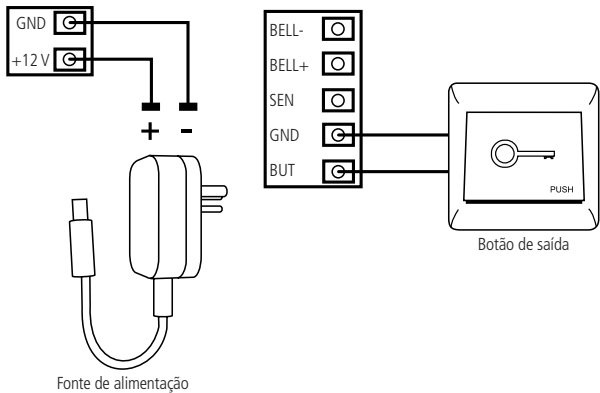
Ligação botão de saída
