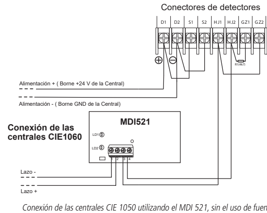
Conexión de las centrales CIE 1050 utilizando el MDI 521, sin el uso de fuentes auxiliares
