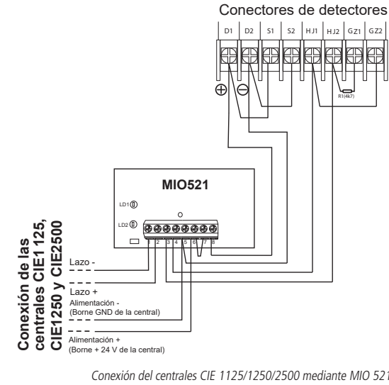
Conexión de las centrales CIE 1125, CIE1250 y CIE2500 mediante MIO 521
