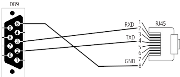
Cabo console
