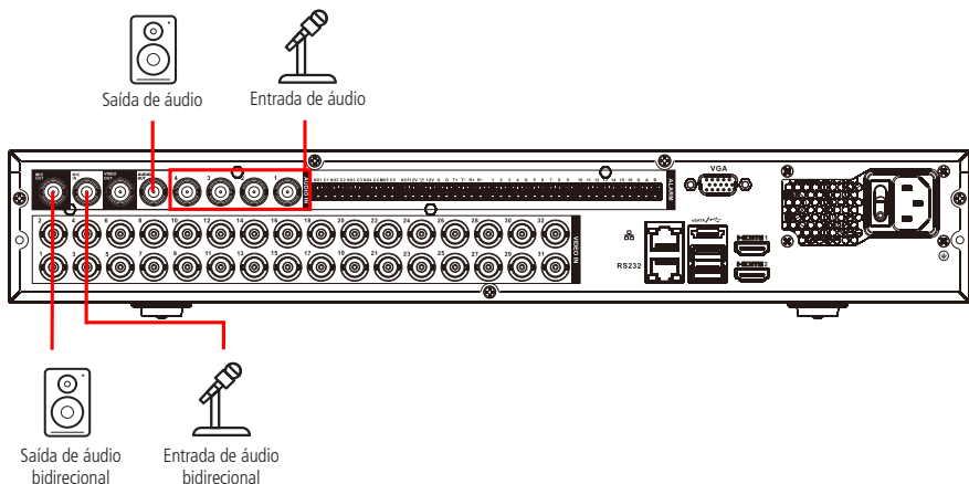
Conexões de áudio MHDX 7132
