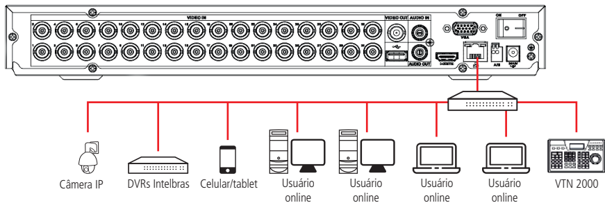
Dispositivo IP MHDX 3132
