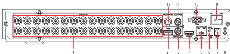
Painel posterior
