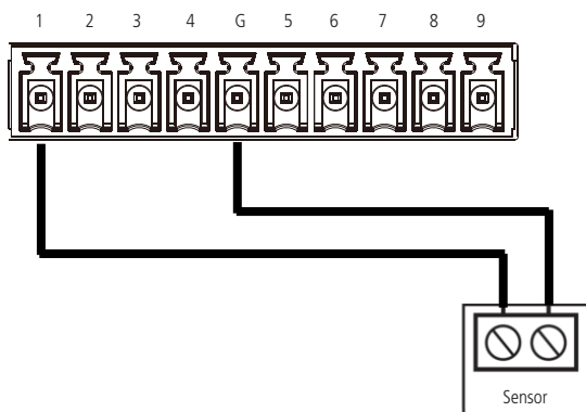
Procedimento para a conexão física dos fios de entrada de alarme
