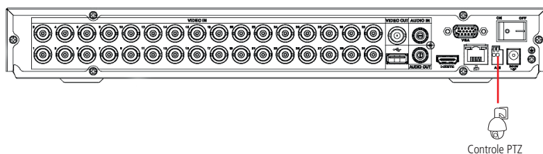
Dispositivos PTZ MHDX 3132
