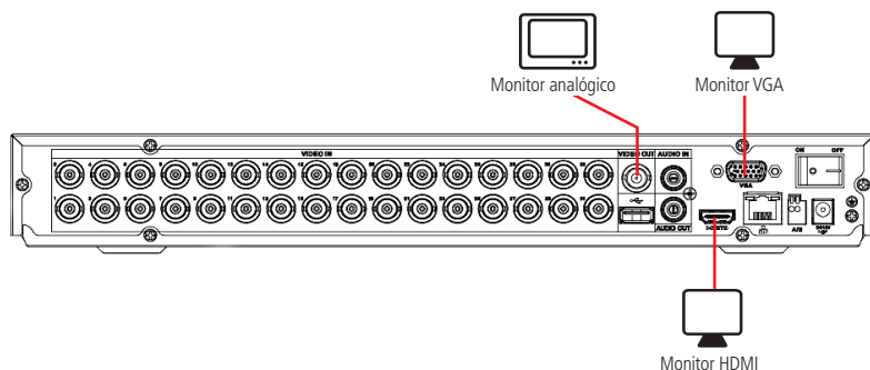
Saídas de vídeo MHDx 3132
