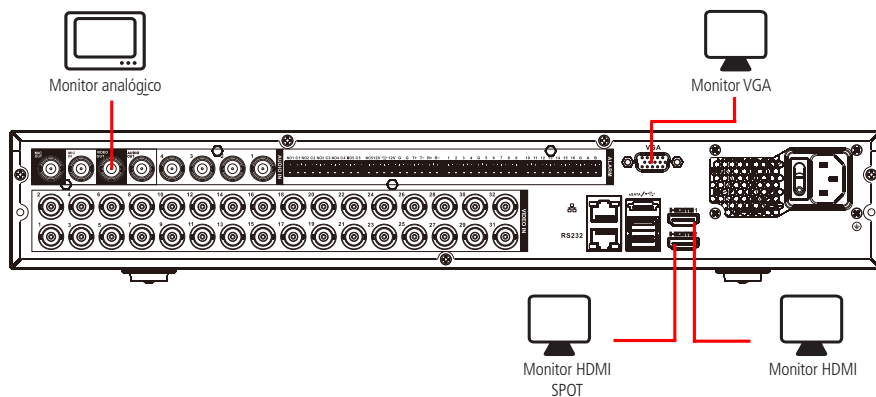
Saídas de vídeo MHDx 7132
