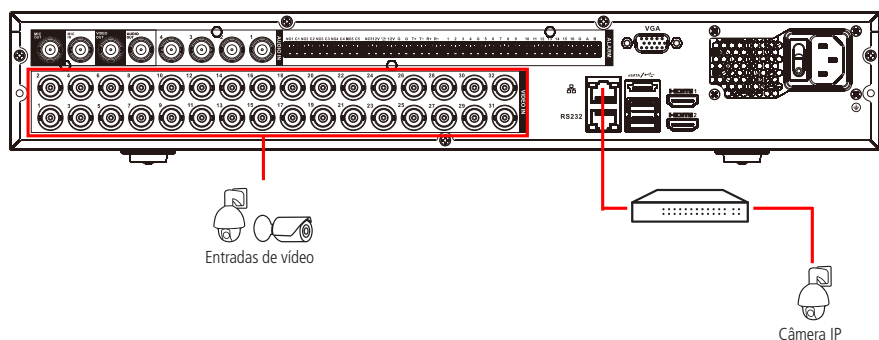
Entradas de vídeo MHDX 7132
