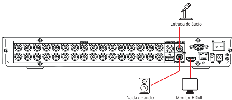
Conexões de áudio MHDX 3132
