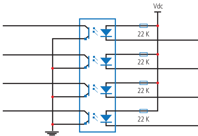
Módulo de entrada de alarme
