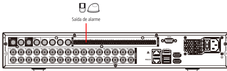
Saída de relé
