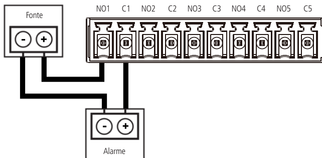
Procedimento para a conexão física dos fios da saída de alarme
