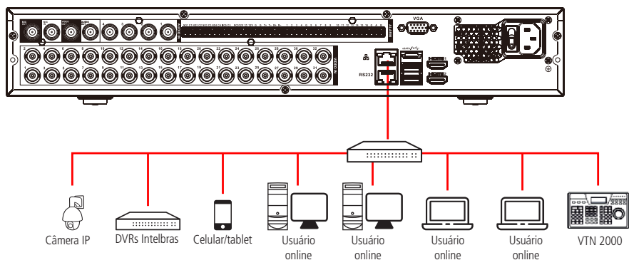
Dispositivo IP MHDX 7132
