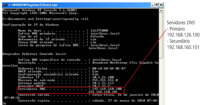
Servidores DNS
