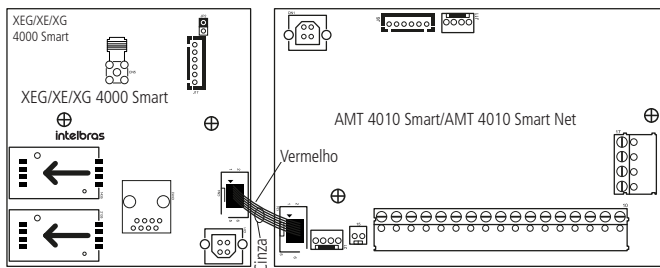
Esquema de ligação módulos de comunicação
