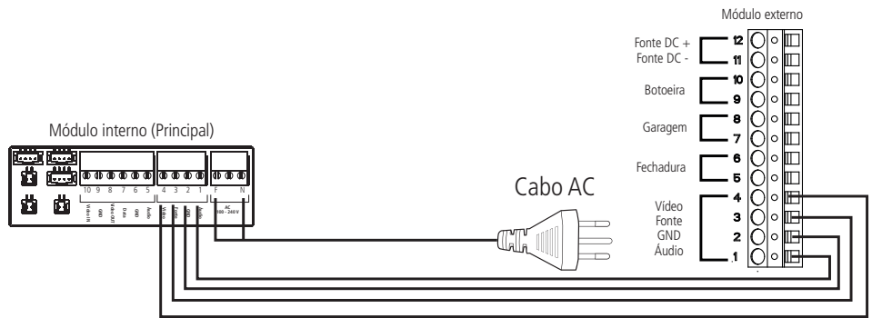
Instalação básica
