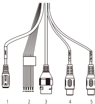
Cabo multifunções VIP 3280 B AL
