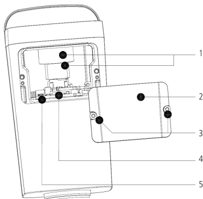
Visão inferior VIP 3280 B AL
