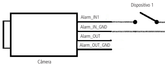
Esquema de entrada de alarme VIP 3280 B AL
