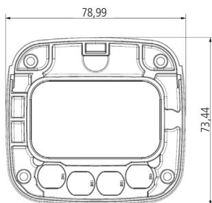
Visão frontal VIP 3280 B AL
