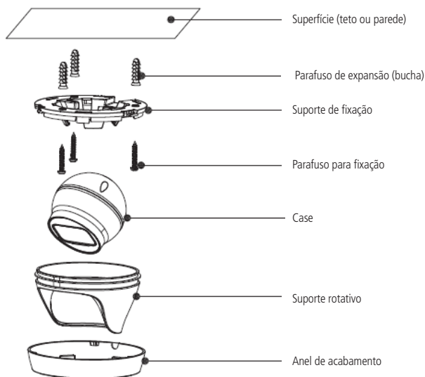
Vista detalhada VIP 1130 D G3 e VIP 1230 D G3
