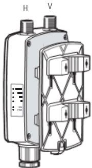
Identificação de polarização da antena
