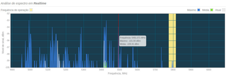
Análise de espectro – Nível de sinal, dBm
