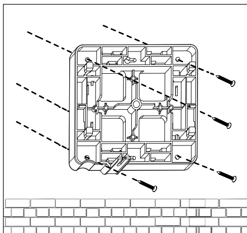
Fixando bracket na parede
