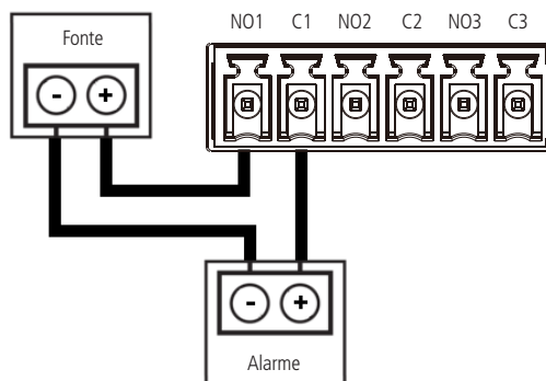
Procedimento para a conexão física dos fios da saída de alarme
