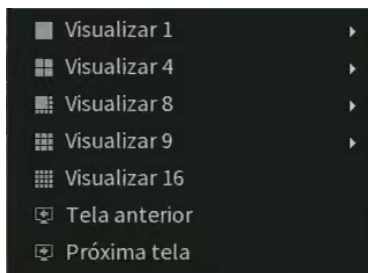
Menu auxiliar
