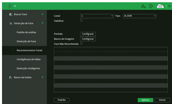
Reconhecimento Facial
