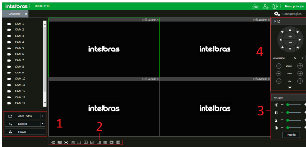
Interface web
