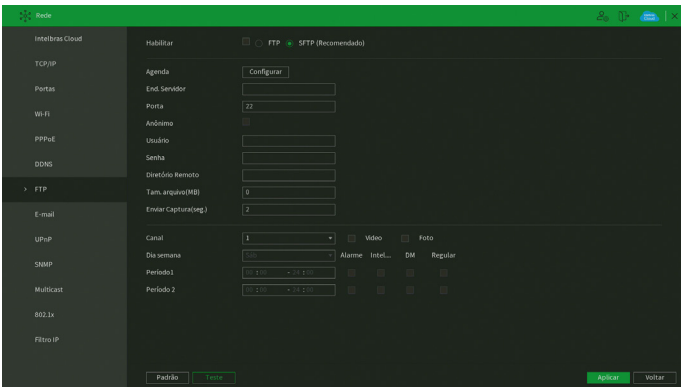
Menu FTP
