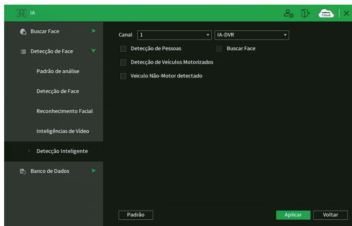
Detecção Inteligente
