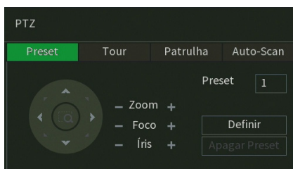
Configurações aux.
