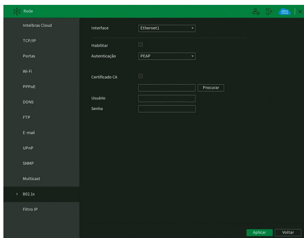
Menu 802.1x
