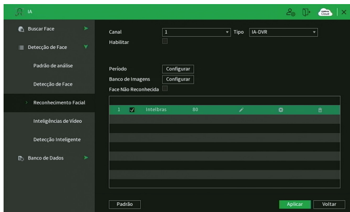
Reconhecimento Facial
