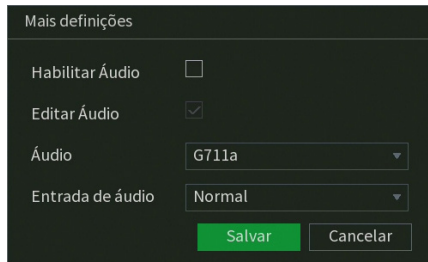
Mais definições
