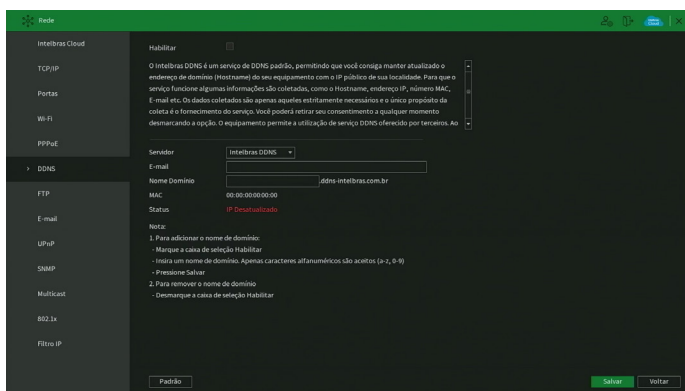
Menu DDNS
