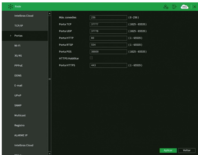
Menu Portas
