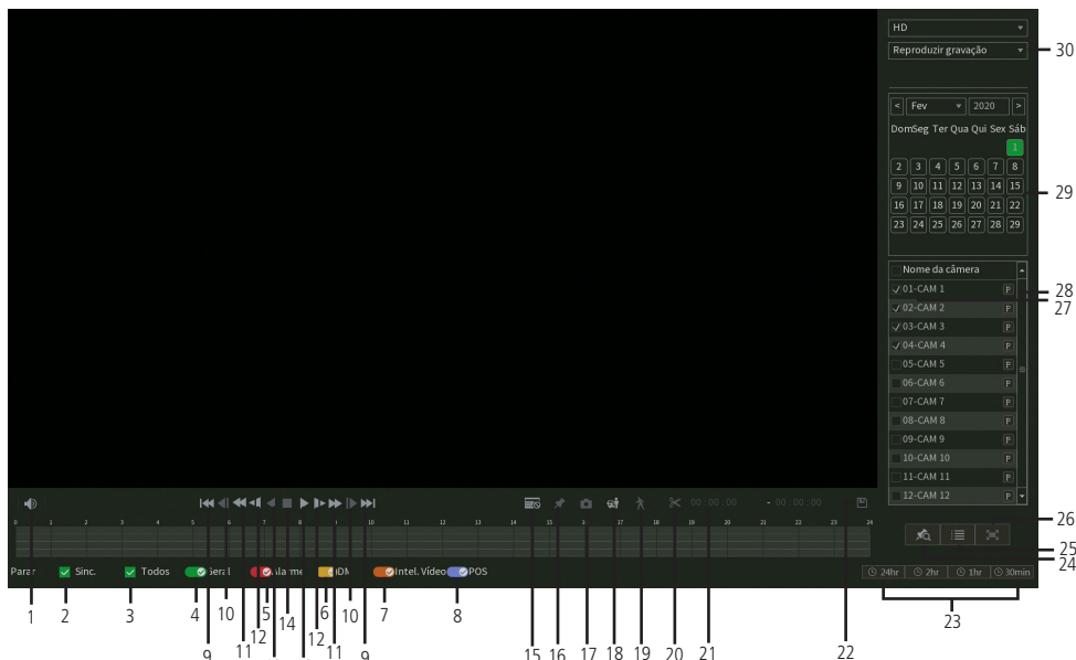
Menu Reproduzir
