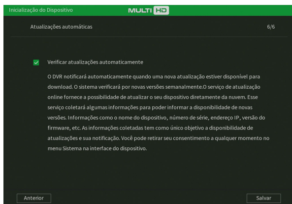
Atualização automática
