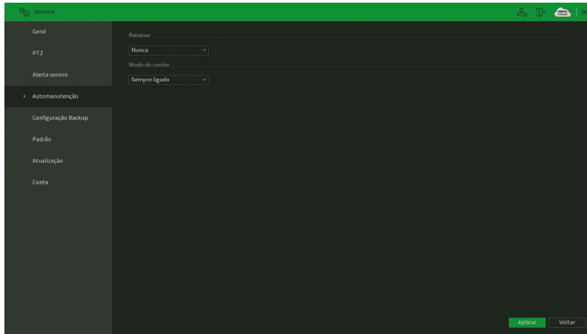
Menu Automanutenção
