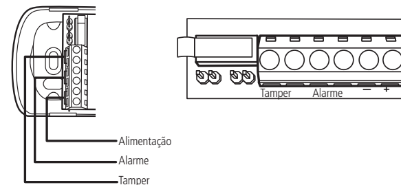
Bloco de terminais
