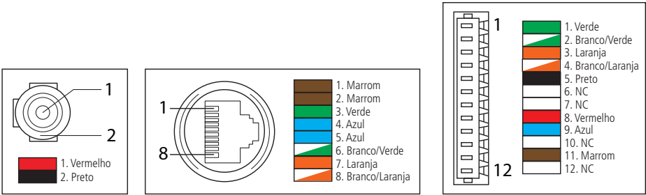
Cabo multifunções VIP 3230 B SL G2 e VIP 3230 D SL G2
