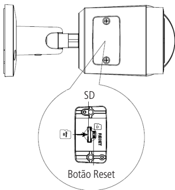
Tampa inferior VIP 3230 B SL G2
