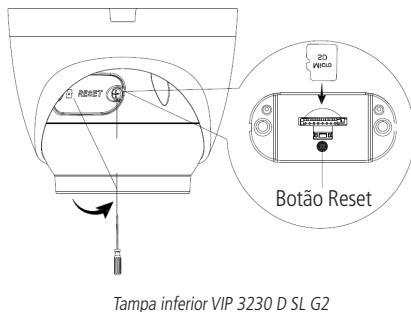
Tampa inferior VIP 3230 D SL G2
