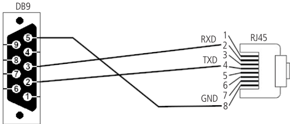
Cabo console
