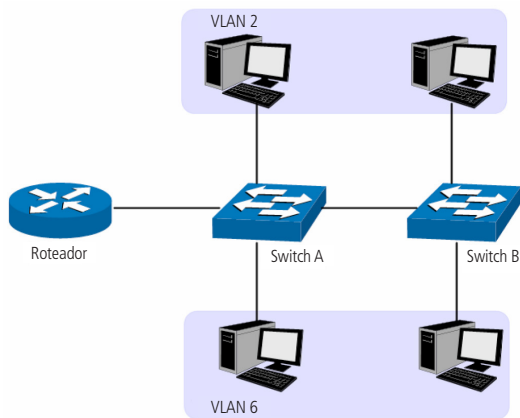
Implementação de VLAN
