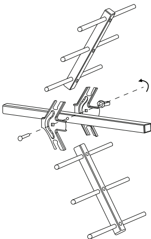
Montagem do refletor
