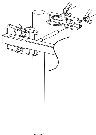
Instalação do suporte de fixação
