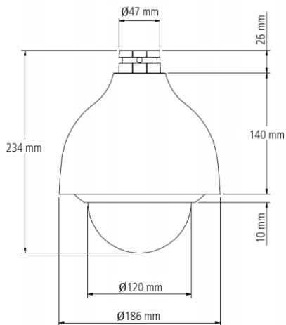
Dimensões da câmera
