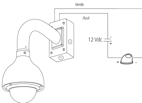
Conexão dos dispositivos de áudio
