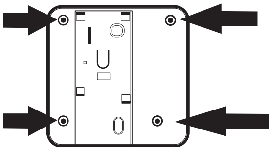
Fixadores do gabinete
