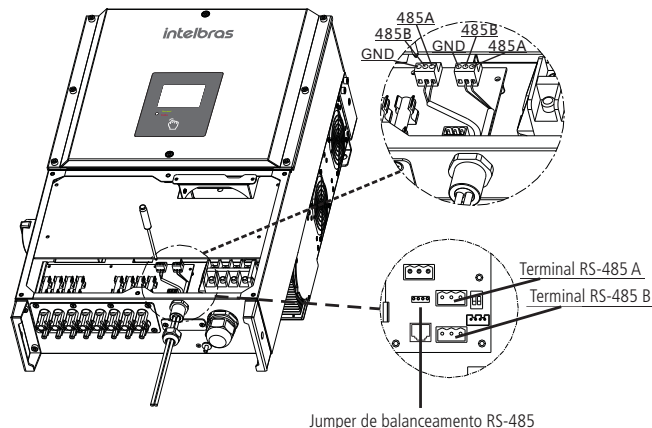
Jumper de balanceamento RS-485
