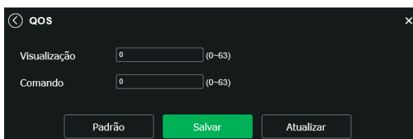
QoS
