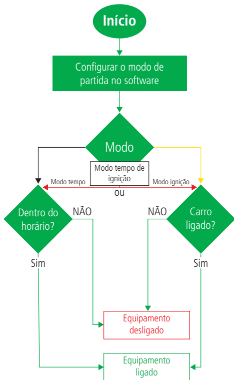
Fluxograma do modo de partida
