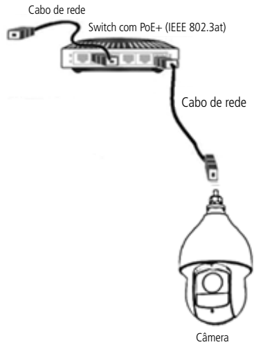
Instalação usando switch PoE+
