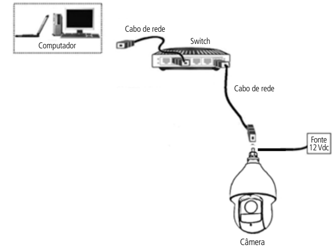
Instalação usando fonte 12 Vdc
