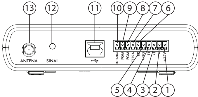
Imagem 04 – Parte traseira do GPRS 1000 UN
