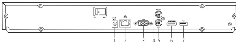
Painel posterior
