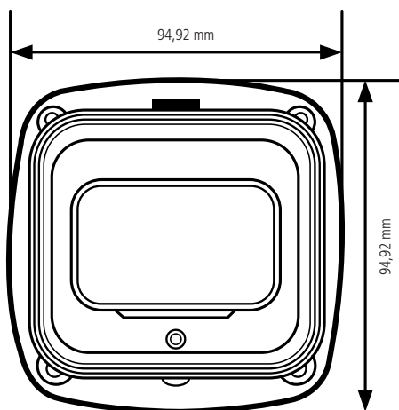
Visão frontal VIP 5450 Z
