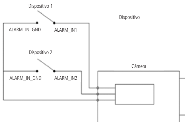
Esquema de entrada de alarme VIP 5450 Z
