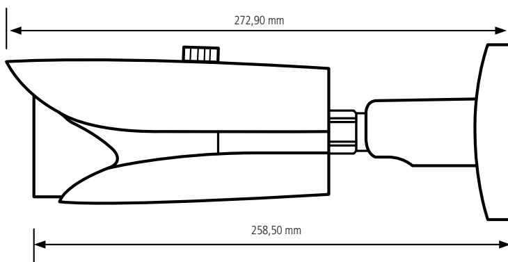
Visão lateral VIP 5450 Z
