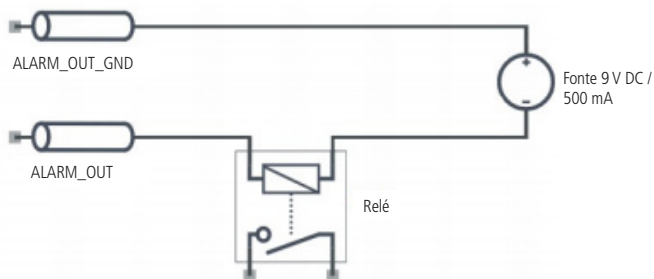
Esquema de saída de alarme VIP 5450 Z
