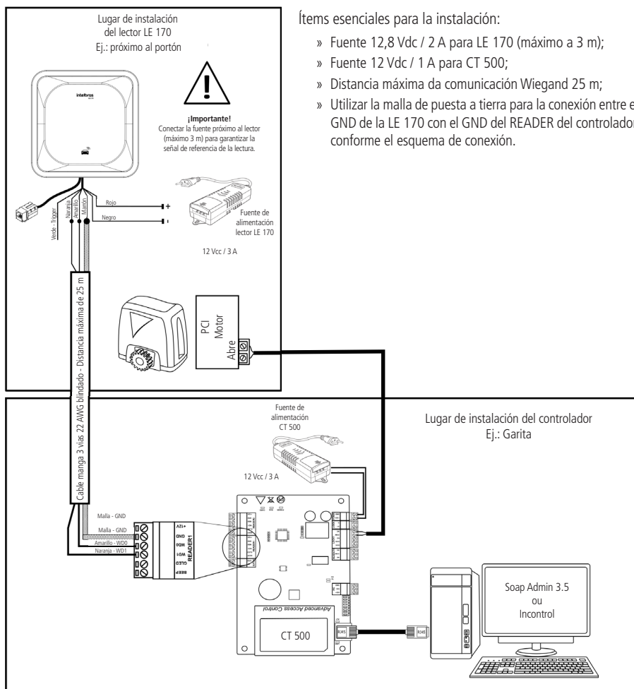
Conexión CT 500 con cable manga blindado
