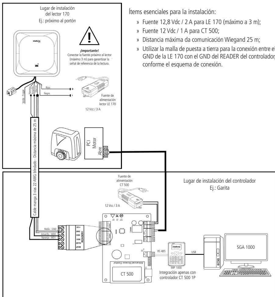
Conexión MIP con cable manga blindado
