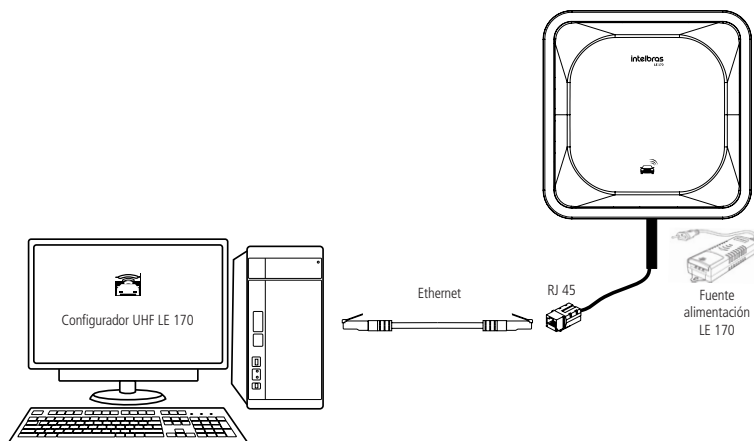
Conector ethernet con la PC
