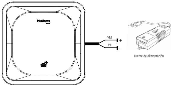
Conexión de la fuente de alimentación
