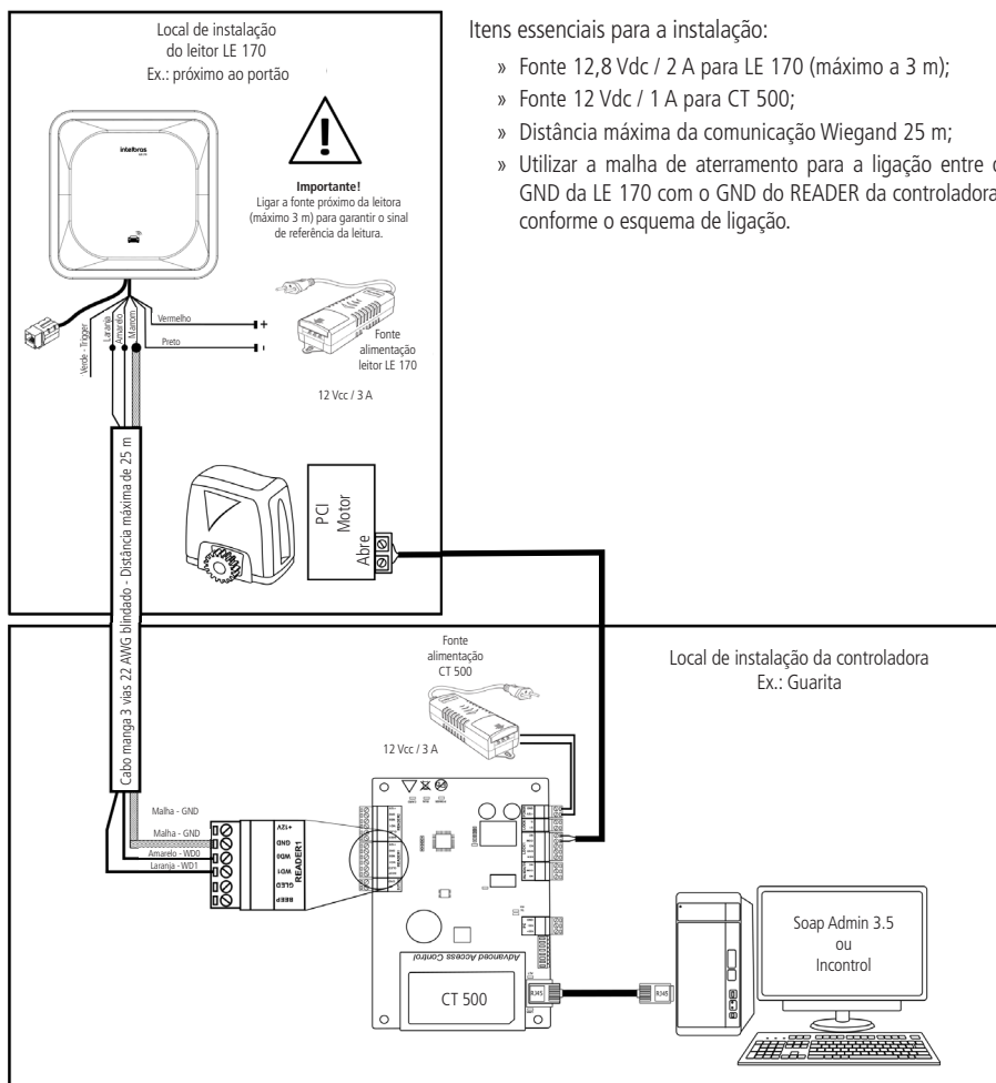
Ligação CT 500 com cabo manga blindado
