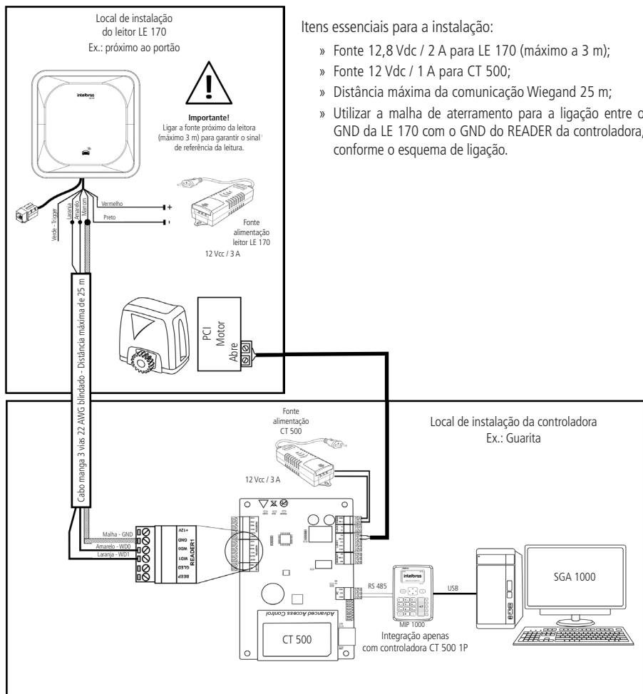
Ligação MIP com cabo manga blindado
