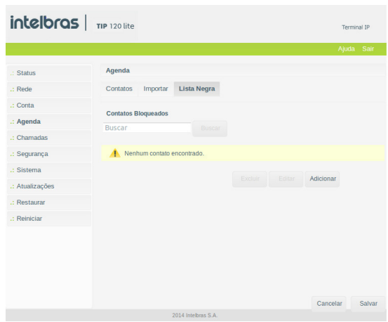
Lista negra
