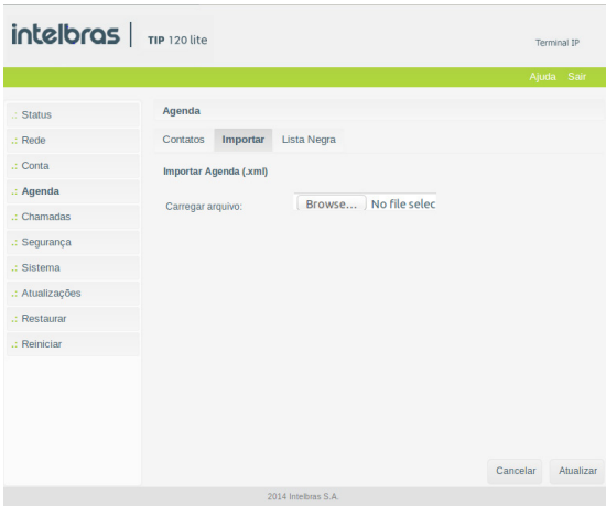
Importar
