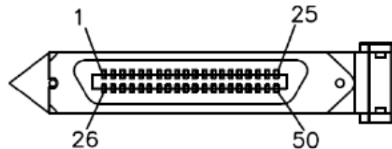
Pinagem Conector Macho
