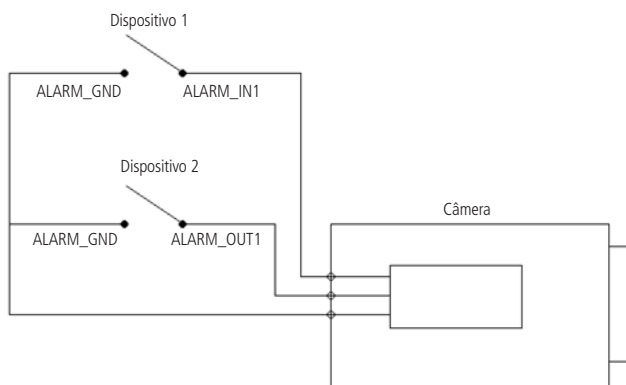
Esquema de entrada e saída de alarme
