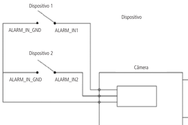
Esquema de entrada de alarme VIP E3250 Z
