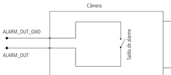
Esquema de saída de alarme VIP E3250 Z
