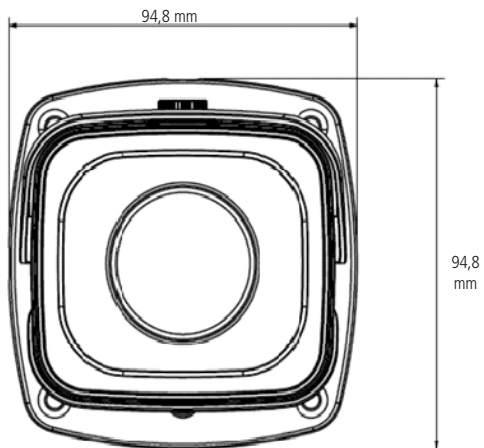
Visão frontal VIP E3250 Z
