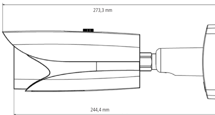
Visão lateral VIP E3250 Z
