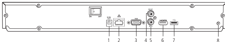
Painel posterior
