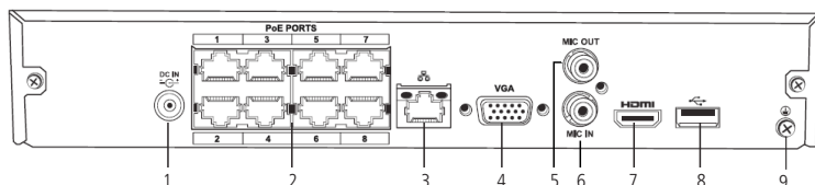
Painel posterior
