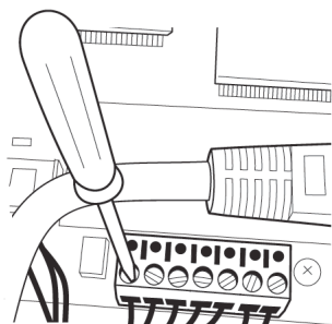
Conexão dos fios no conector CN7
