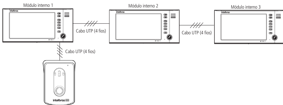
Instalação com 3 módulos internos e 1 módulo externo
