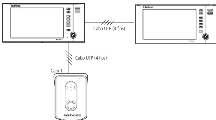
Instalação com 2 módulos internos e 1 módulo externo
