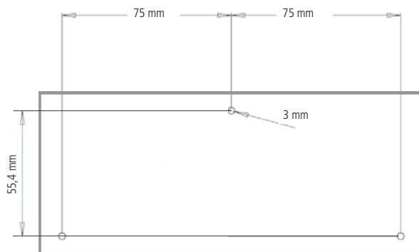
Gabarito de fixação
