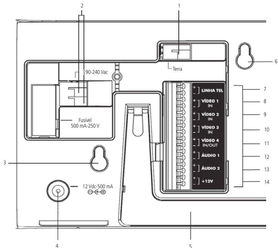
Vista posterior
