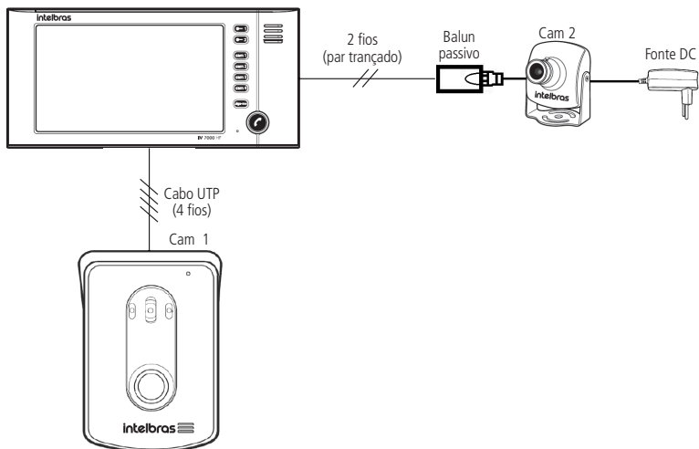
Instalação com 1 câmera extra
