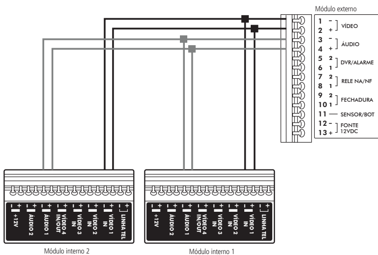
Conexão com 2 módulos internos e 1 módulo externo
