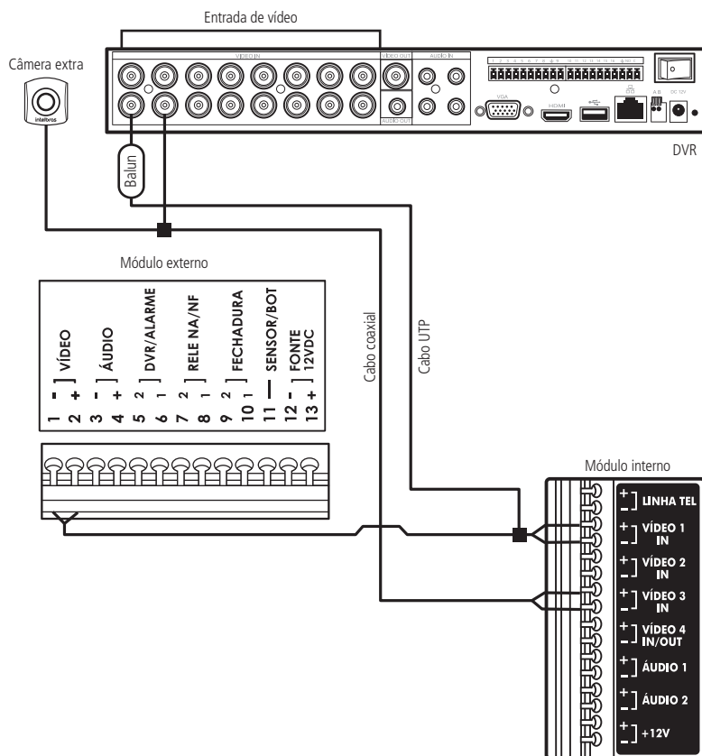
Ligação de vídeo paralela com DVR
