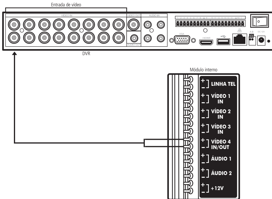
Gravar imagens do videoporteiro no DVR
