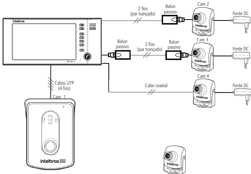
Instalação com 3 câmeras extras
